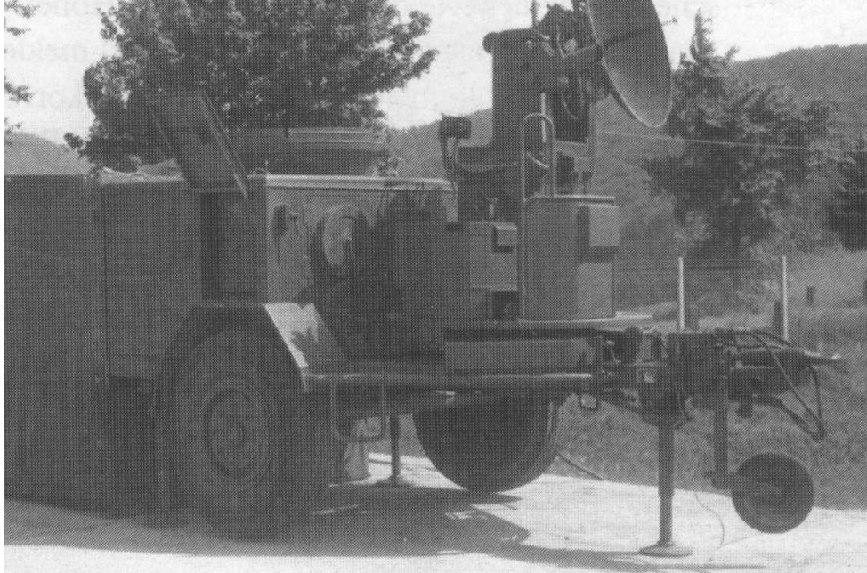
Höhenwindradar D (DEISWIL) IV Nutzungszeit 1962-1967
